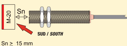
APERTURA CONTATTO CON IL SUD DEACTIVATED BY THE SOUTH POLARITY
