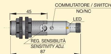
MODELLI CON CONNETTORE H MODELS WITH H PLUG
