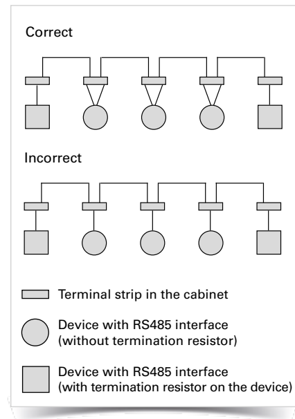
Fig.: Modbus configuration
