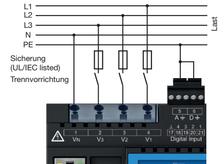
Abb. Anschlussbeispiel „Spannungsmessung“.
