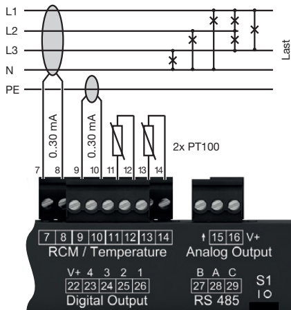
Anschlussbeispiel Multifunktionskanäle für die Differenzstrom- und Temperaturmessung
