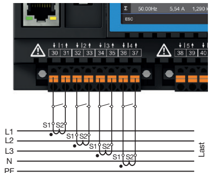
Abb. Anschlussbeispiel „Strommessung“.
