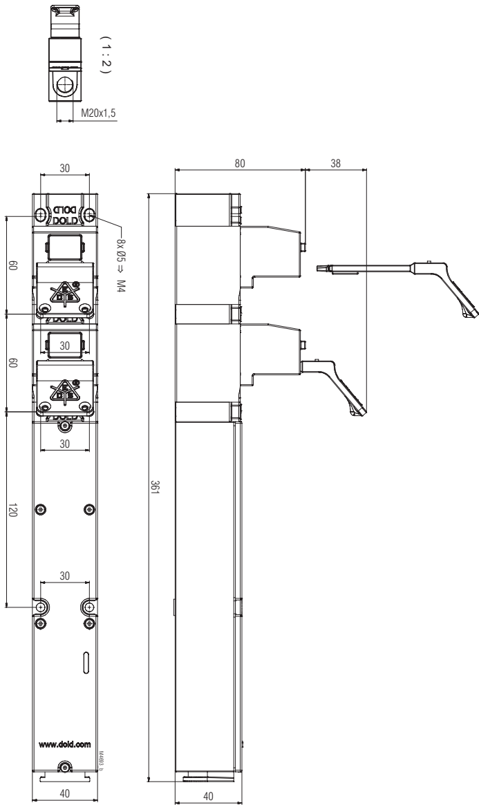
YRH11M Tolérances générales \pm 2\%
