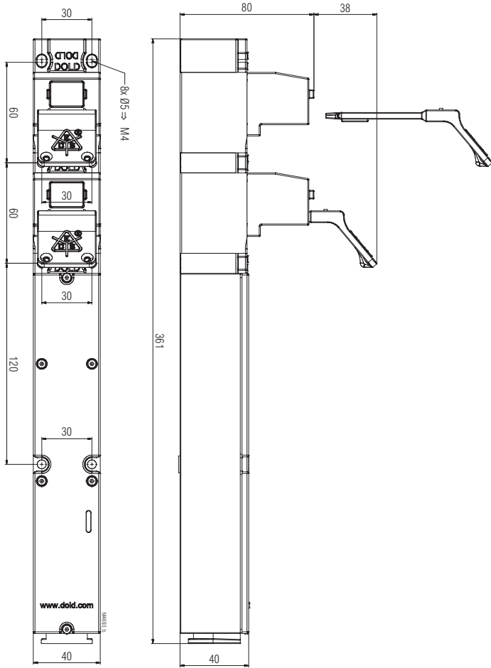
YRX11M/K Freimaßtoleranzen \pm 2\%
