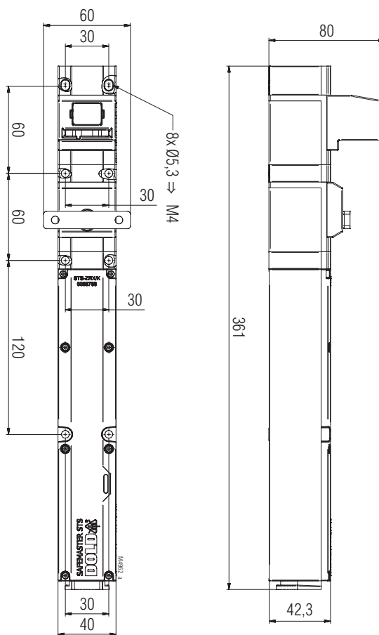
YRXK01M/K Freimaßtoleranzen ± 2%
