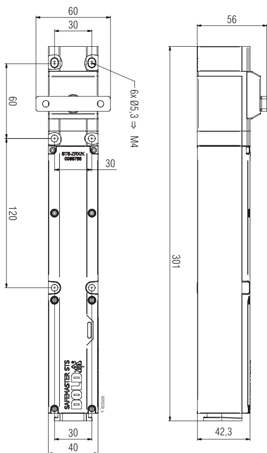
YRXKM/K Freimaßtoleranzen ± 2%
