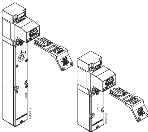
Steckschlüssel gezogen mit einem ZRH01M
