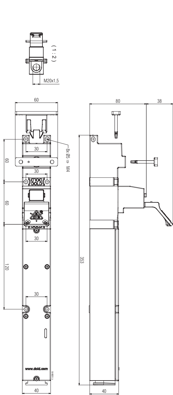
Abbildung: YRX10A Freimaßtoleranzen ± 2%
