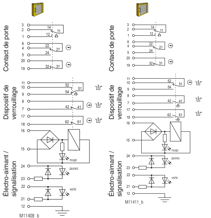
Fig. 1 : Gâche à l'état activé: Solénoïde enclenché, clé insérée
