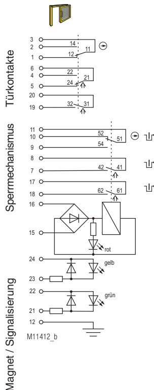
Bild 1: Zuhaltung im aktivierten Zustand: Magnet verriegelt, Schlüssel gesteckt
