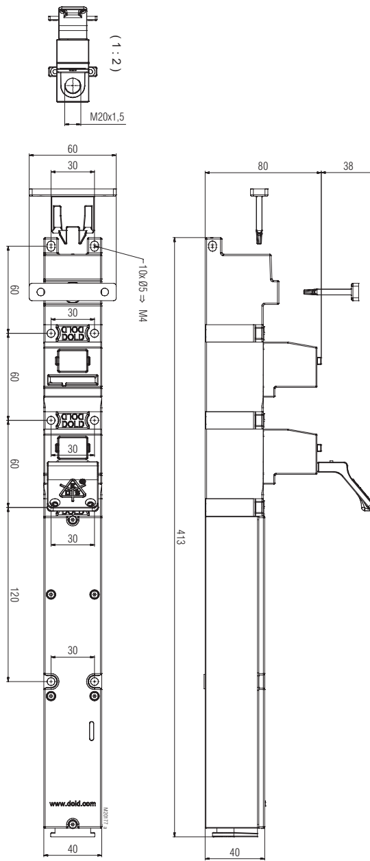
Abbildung: YRX11A Freimaßtoleranzen ± 2%
